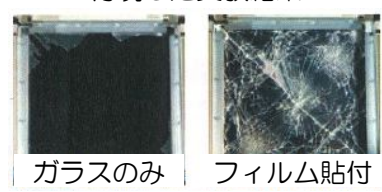
地震で窓枠がゆがんだ状態を再現した実験結果
